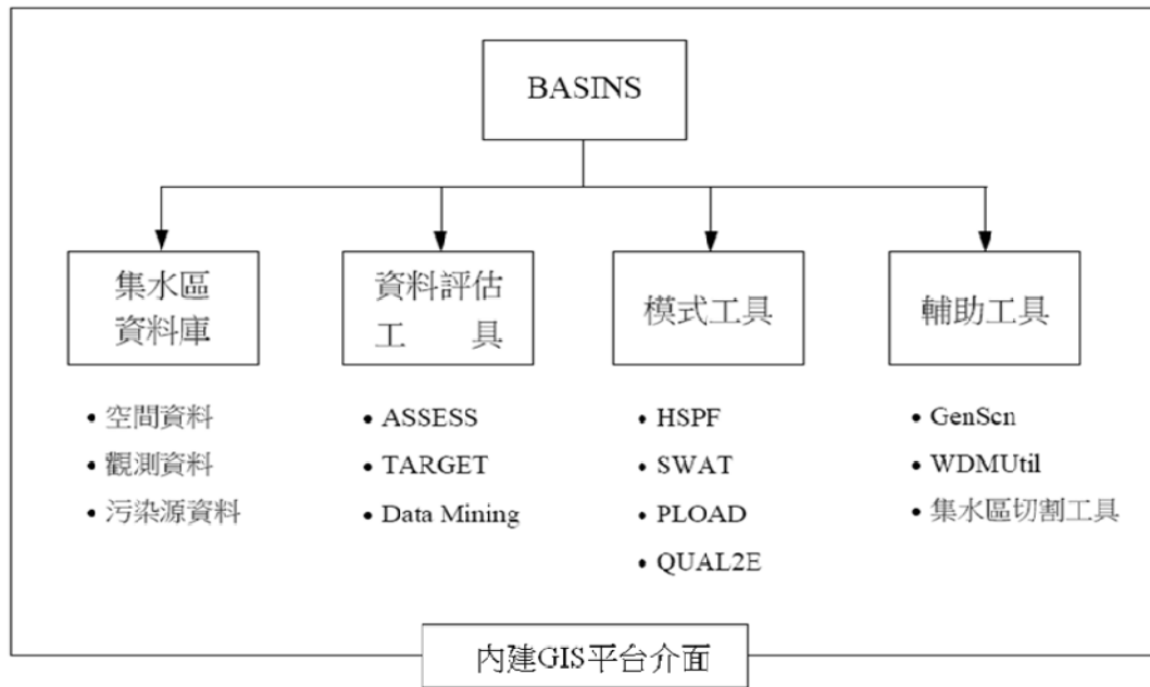
圖2 BASINS架構圖
