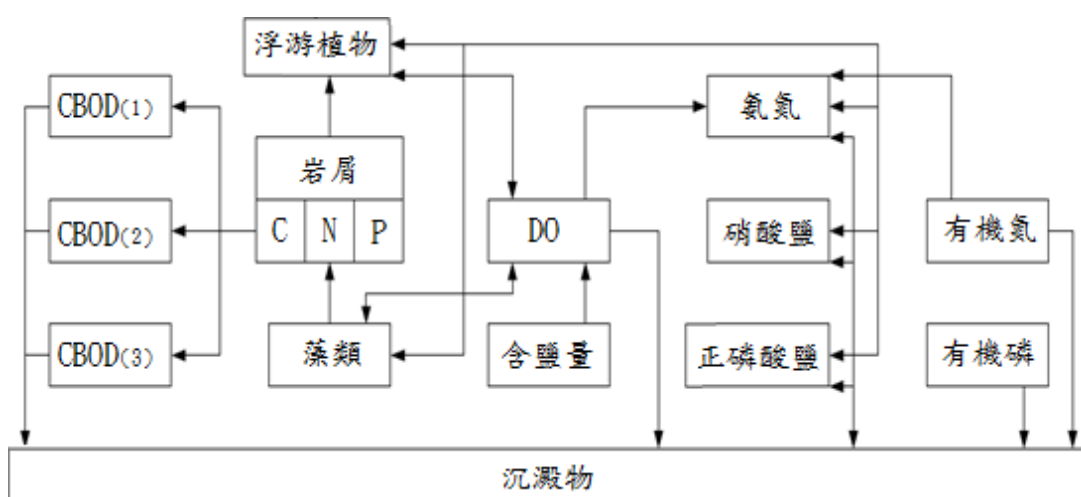
圖 1 EUTRO 模組基本架構
